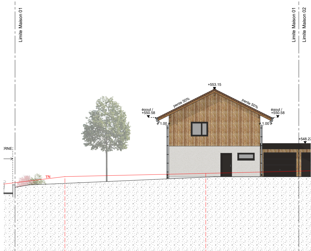
FACADE NORD
